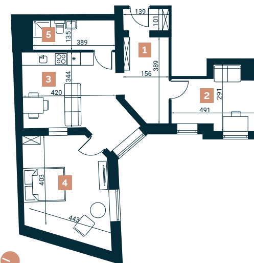
Rzut lokalu nr 55+56
