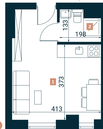
Rzut lokalu nr 23
