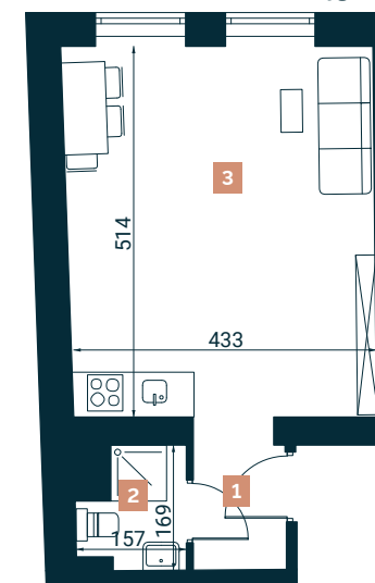
Rzut lokalu nr 28
