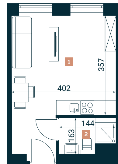
Rzut lokalu nr 29
