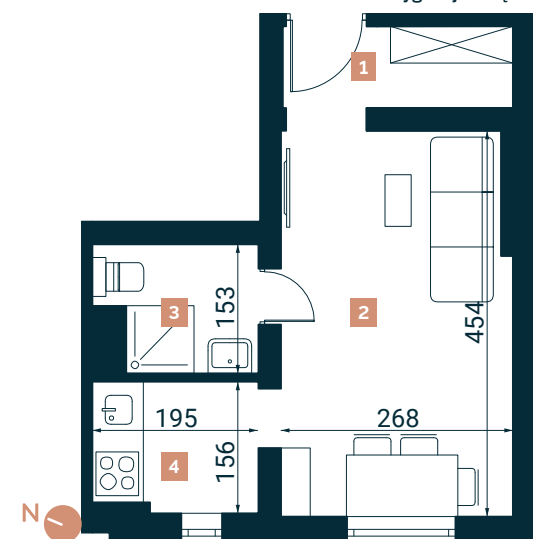
Rzut lokalu nr 30
