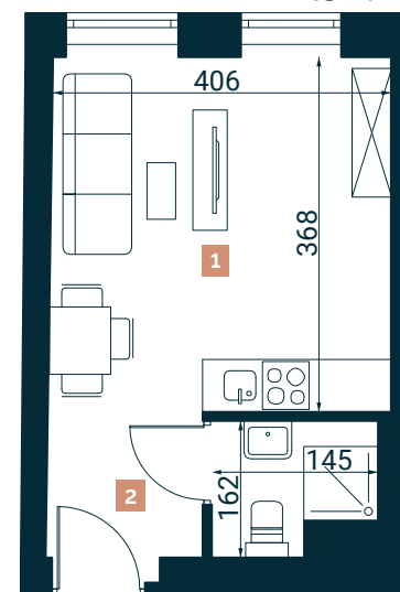
Rzut lokalu nr 40
