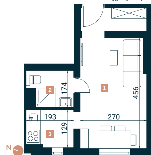
Rzut lokalu nr 51
