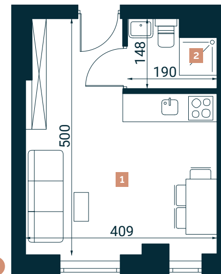
Rzut lokalu nr 9
